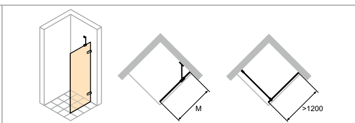
Rechtsbefestigung
