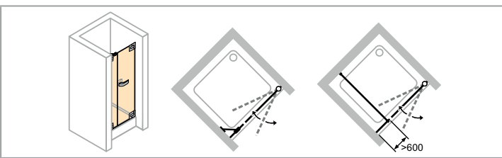
Rechtsbefestigung
