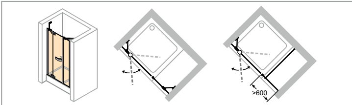
Linksbefestigung
